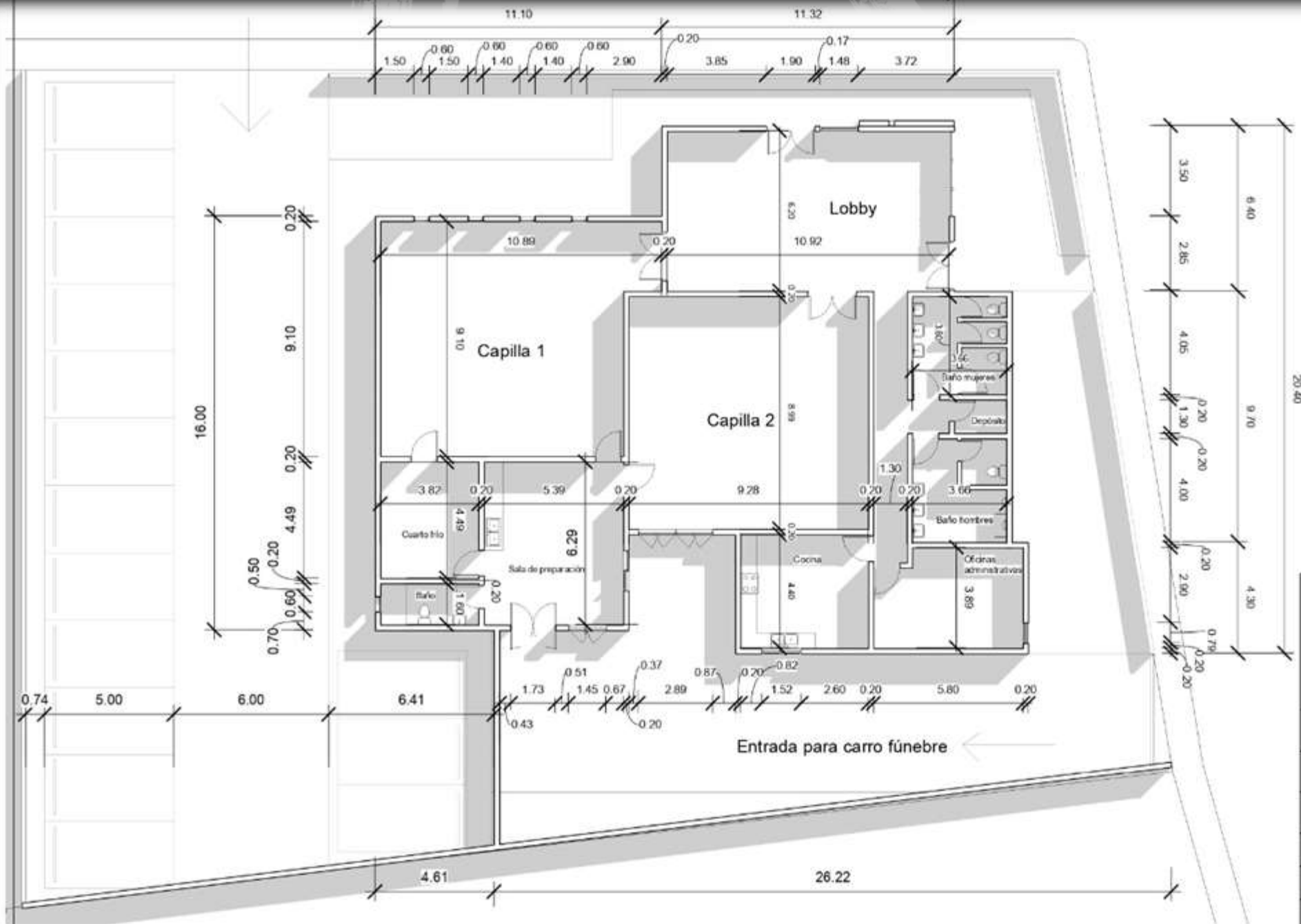
Planta dimensionada
